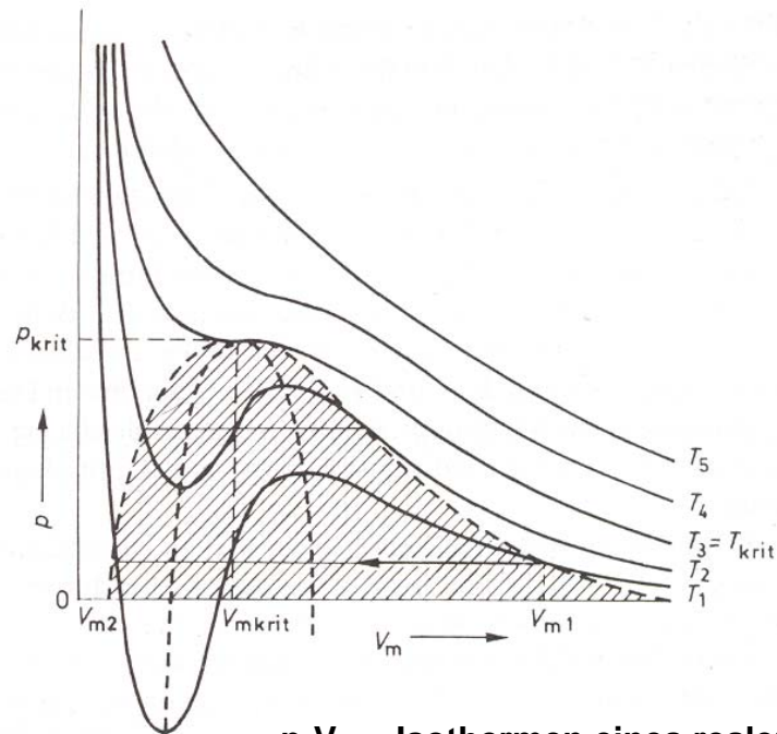
p - V_m – Isothermen eines realen Gases mit schraffiertem Nassdampfgebiet und horizontalem Verlauf von T_{\text{krit}} im kritischen Punkt
