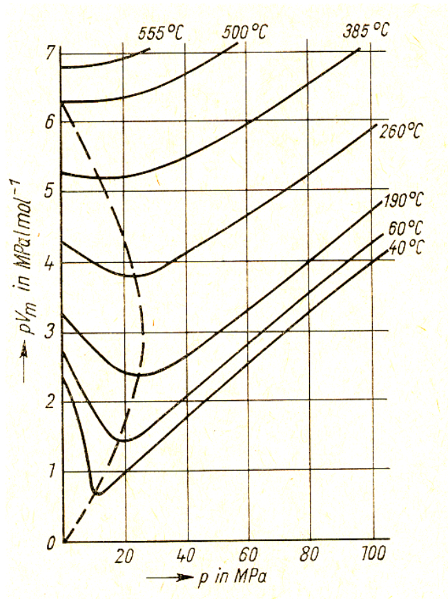
pV_m , p – Isothermen von \text{CO}_2 Boyle-Temperatur: 773\text{ K}
