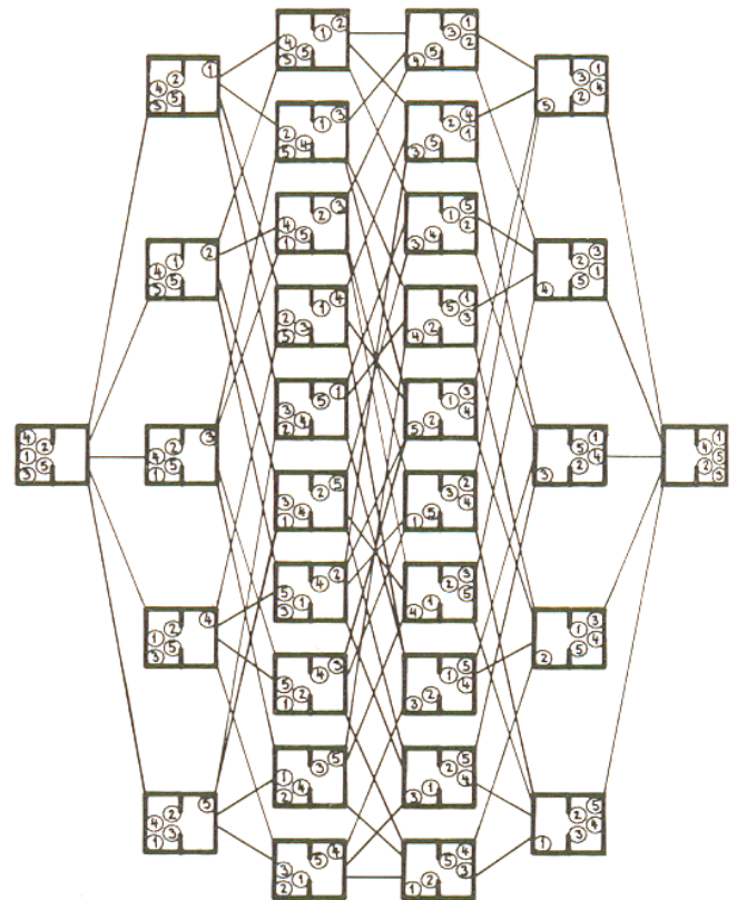
Abb. 5.46. Bei fünf Teilchen überwiegt die gleichmäßige Verteilung noch viel stärker
