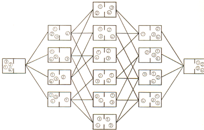
Abb. 5.45. Schon bei vier Teilchen ist eine gleichmäßige Verteilung über beide Hälften eines Volumens viel wahrscheinlicher als eine ungleichmäßige
