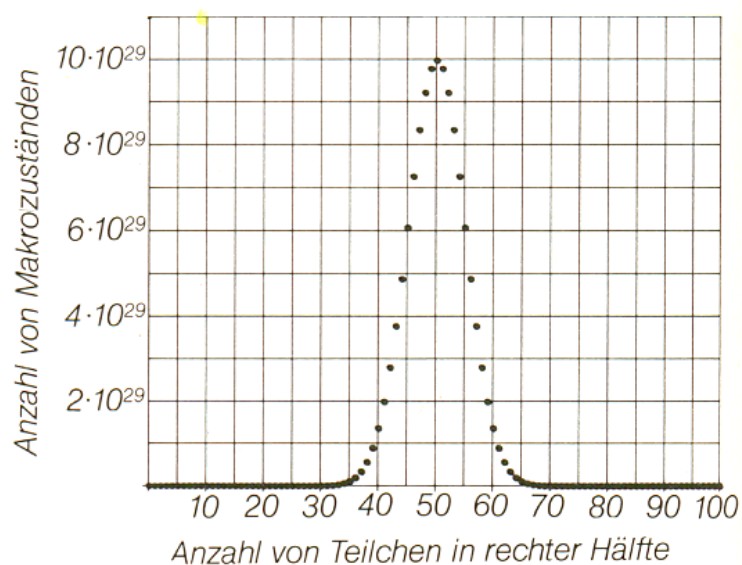
Abb. 5.47. Wahrscheinlichkeiten der Verteilungen von 100 Teilchen über zwei gleiche Teilvolumina
