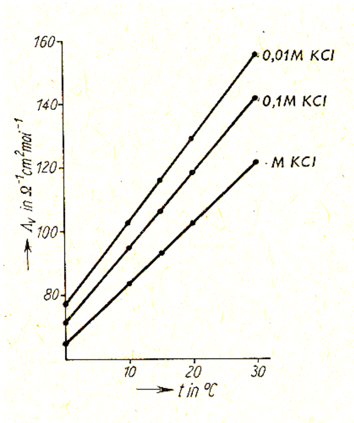
Temperaturabhängigkeit der molaren Leitfähigkeit \Lambda_m (© Näser, 19. Aufl., 1990)
