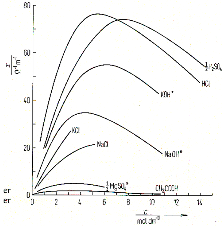
Spezifische Leitfähigkeit \kappa als Funktion von c bei 291 K (© Wedler, 4. Aufl., 1997)
